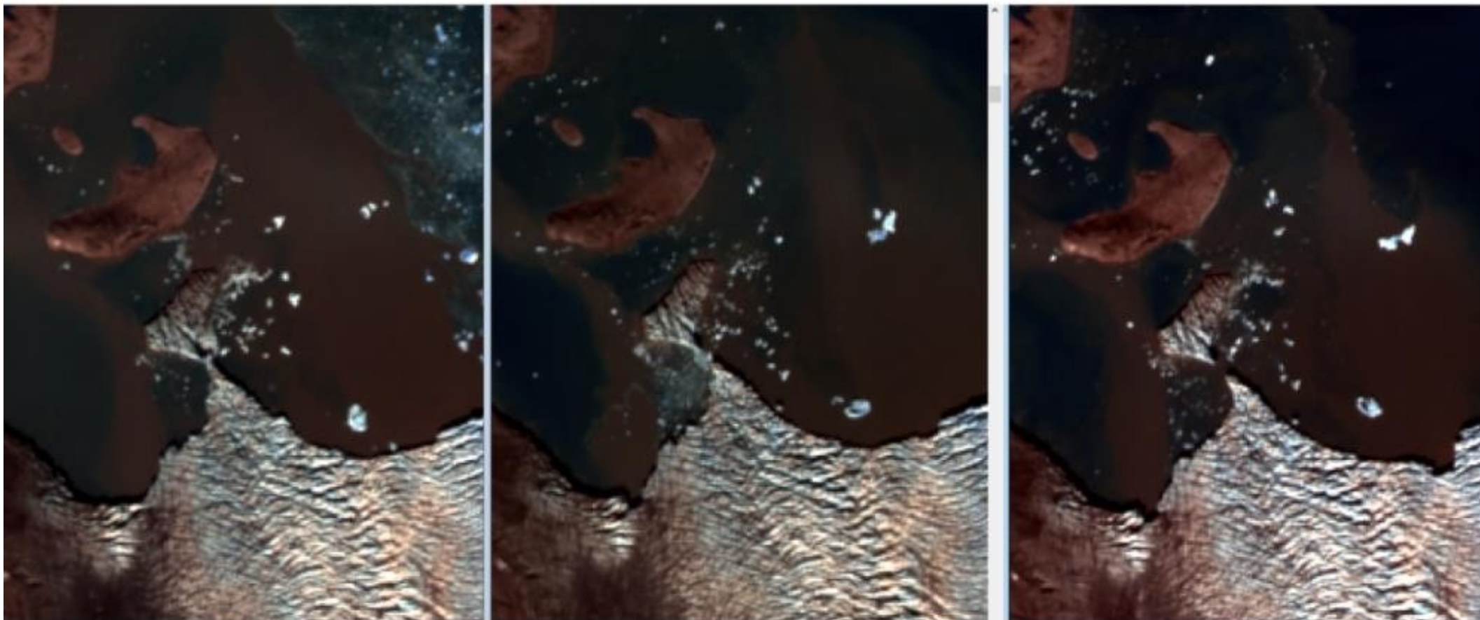
Образование нового острова. 05.07.2020 (слева), 09.07.2020 (в центре) и 11.07.2020 (справа). Сентинель-2. Коперник.
